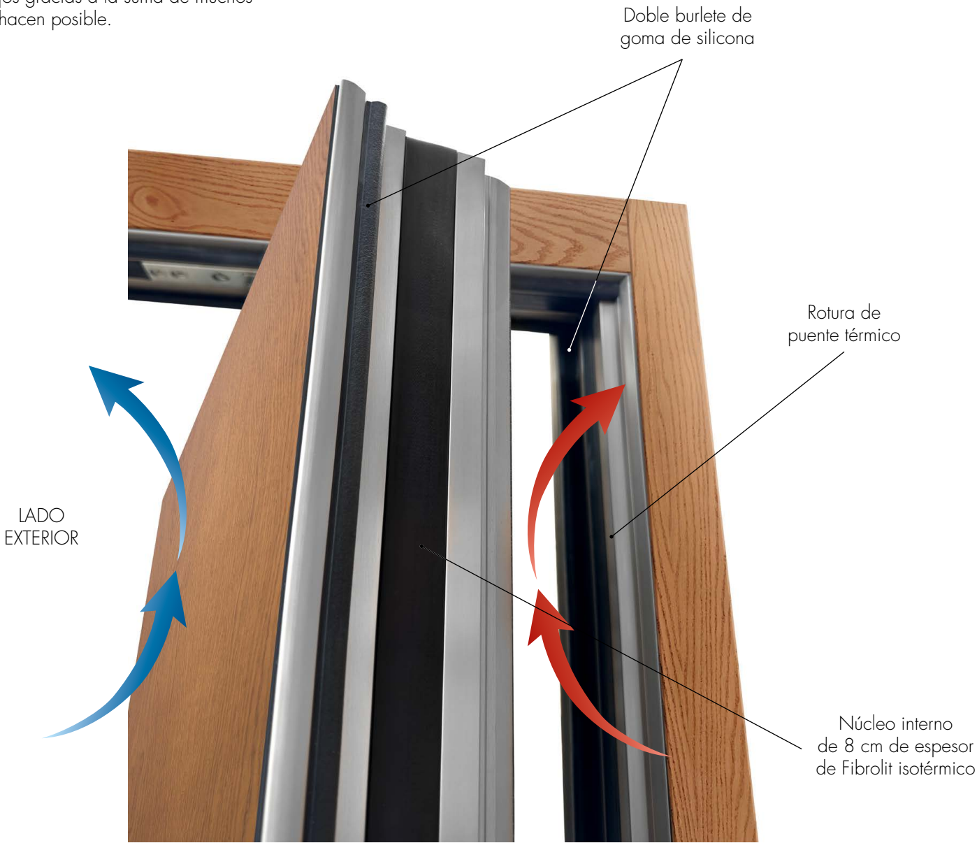
NUEVO BASTIDOR DE ESTRUCTURA METÁLICA
